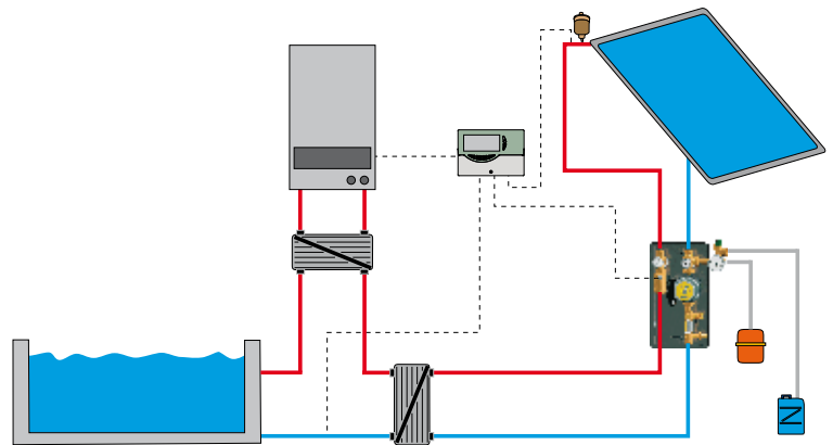
Schema di riferimento Reference schematic
